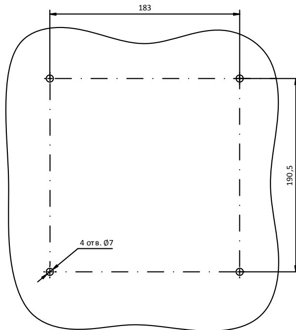
Монтажные отверстия
