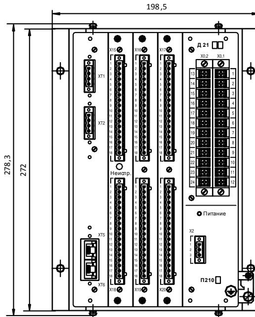
Монтажные отверстия
