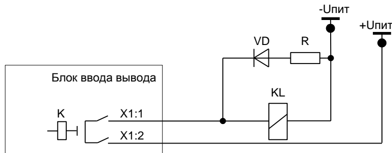
Рисунок 1.3 – Пример подключения промежуточного реле
