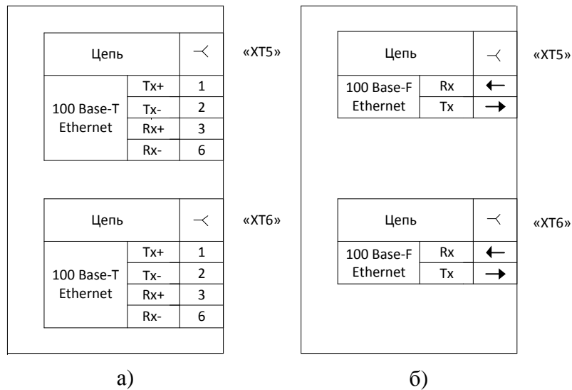
Рисунок Г.2 – Порты связи Ethernet
