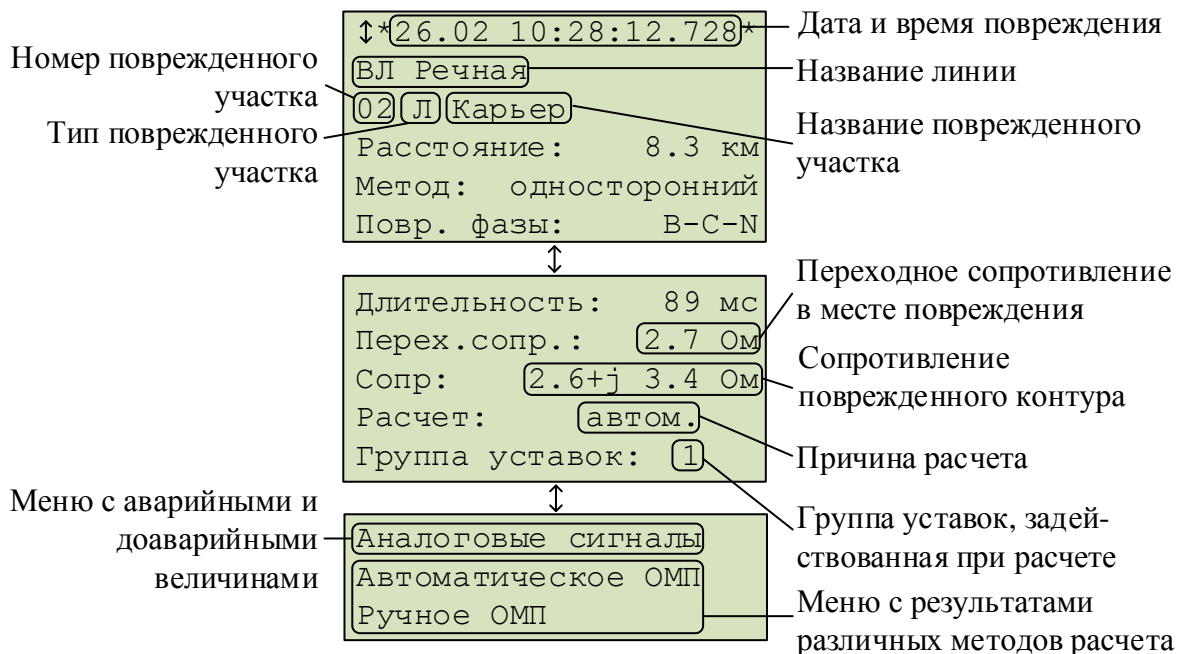
Рисунок 2.2 – Пример отчета ОМП при КЗ в зоне
