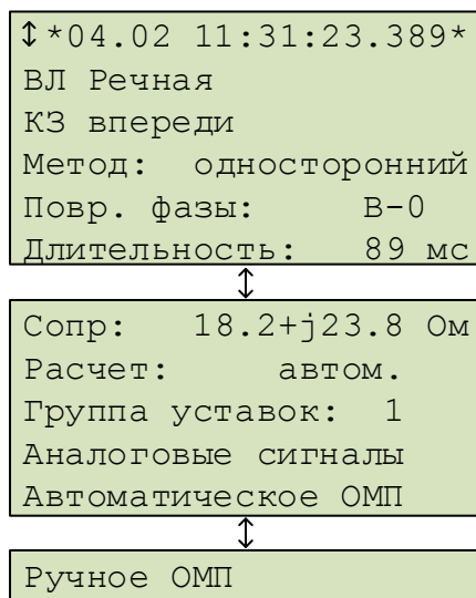
Рисунок 2.3 – Пример отчета ОМП при КЗ впереди
